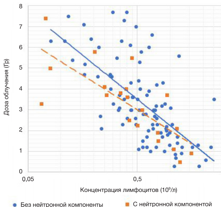
Рис. Зависимость дозы облучения (Гр) от численности лимфоцитов ( \times 10^9/\text{л} ) на 2-е сутки после облучения. Маркерами показаны исходные данные (по отдельности для групп с гамма- и гамма-нейтронным излучением), линиями — наблюдаемая тенденция
